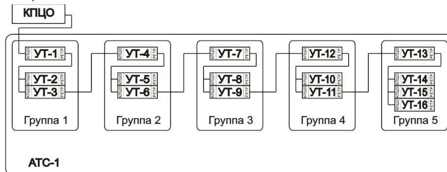
Рисунок 5.13. Группы устройств в рамках одной логической АТС
